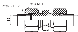
美制 JIC 外螺纹 74° 外锥 JIC MALE 74° CONE
